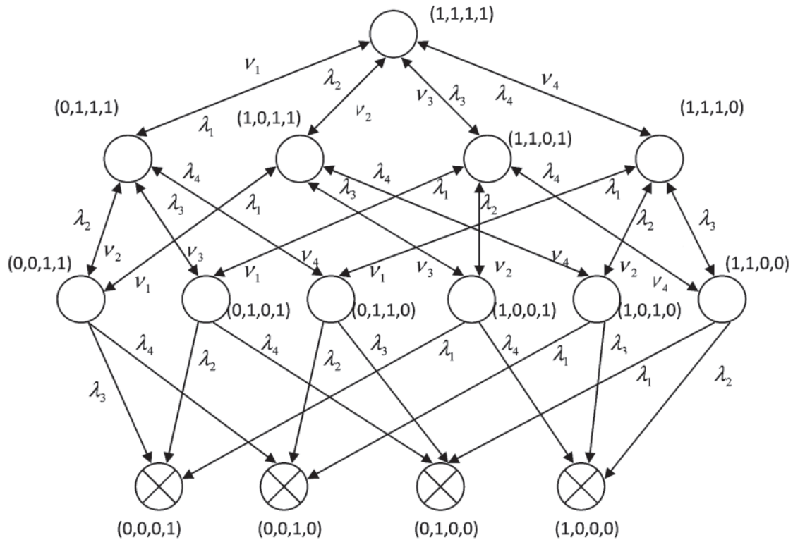
Рис. 2. Граф состояний программной архитектуры с динамической структурой
